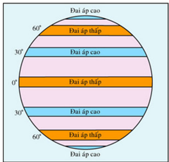
Các đai khí áp trên Trái Đất
