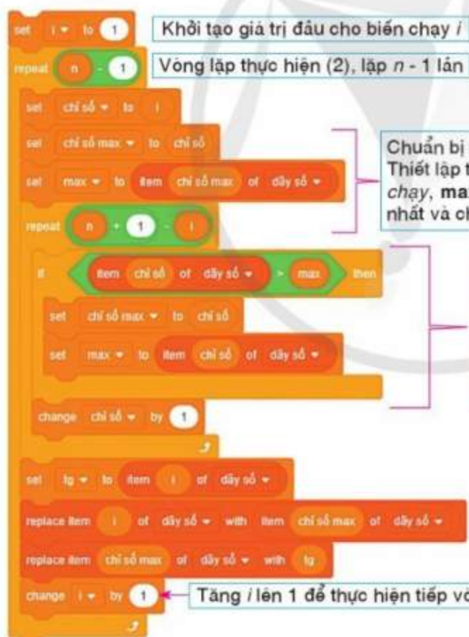
Hình 8. Đoạn chương trình thực hiện chương trình sắp xếp chọn
