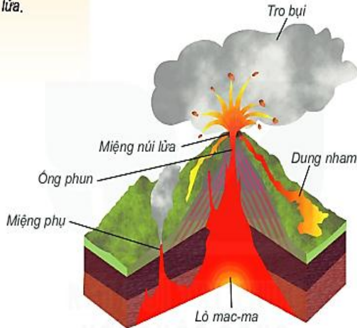
Hình 1. Cấu tạo và hoạt động của một núi lửa
