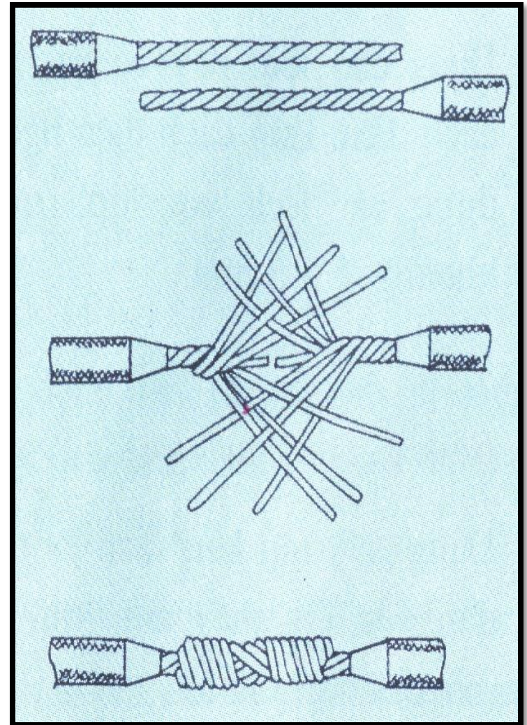
Hình 5.6 Nối nối tiếp dây dẫn lõi nhiều sợi
