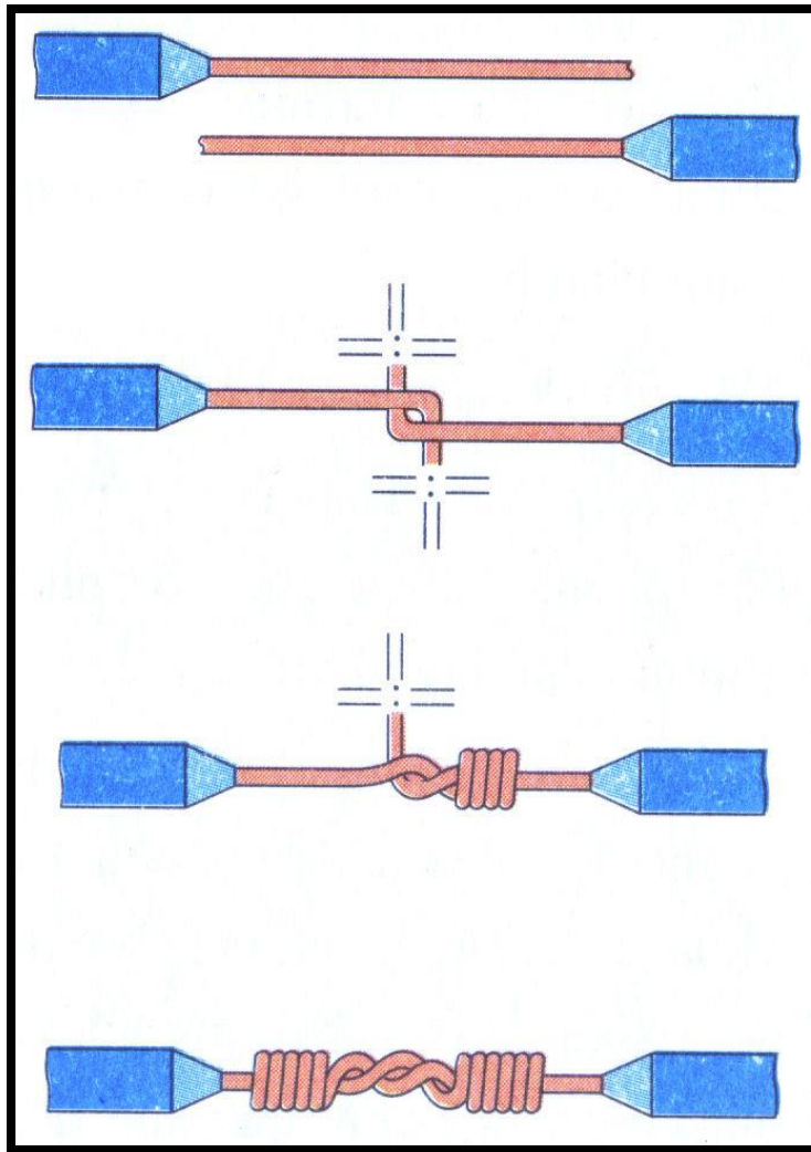
Hình 5.5. Nối nối tiếp dây dẫn lõi 1 sợi
