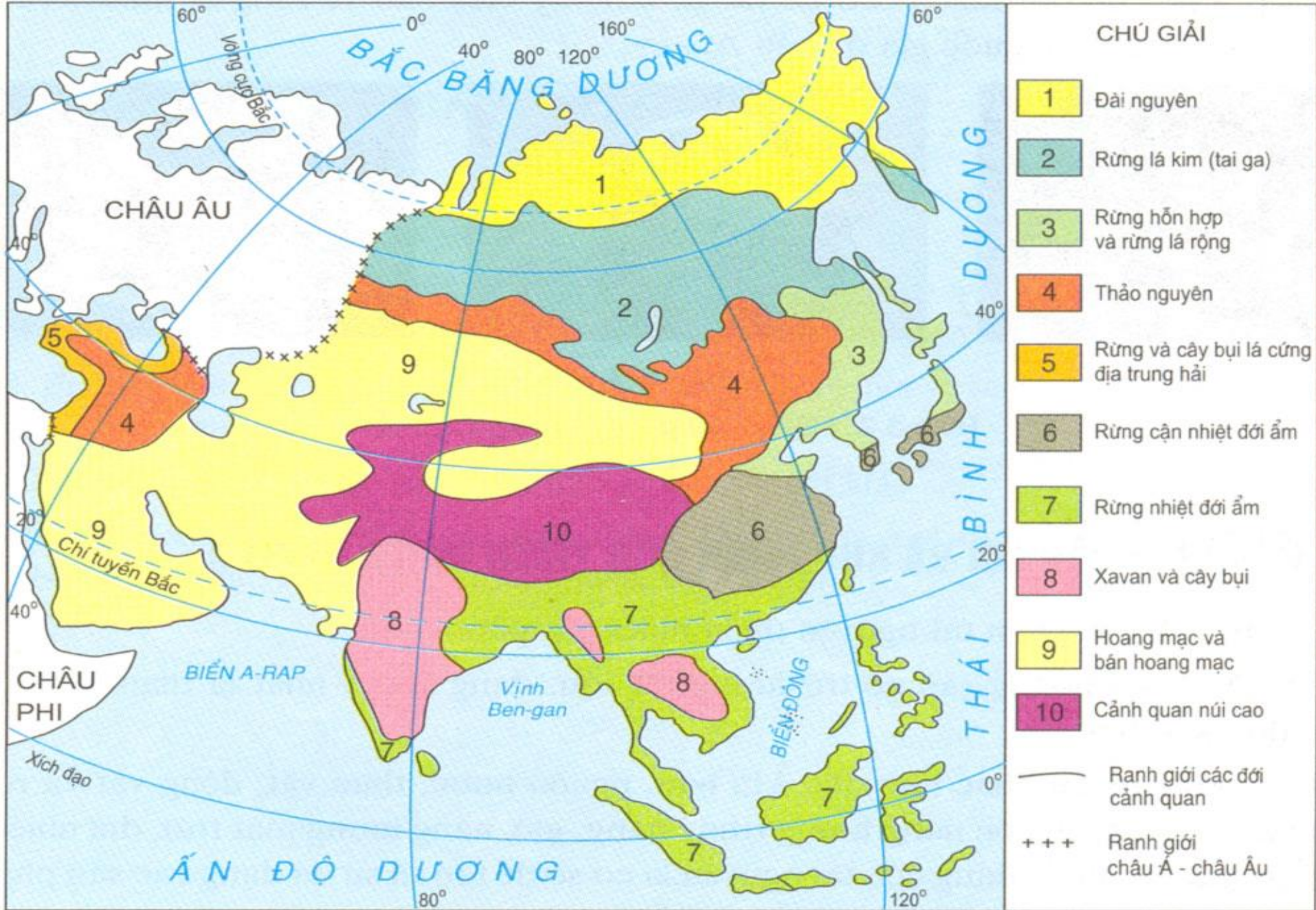
Lược đồ các đới cảnh quan Châu Á
