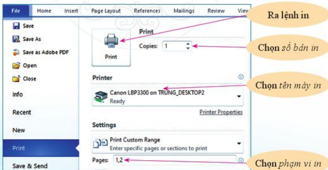
Hình 5. Các tùy chọn in ấn
